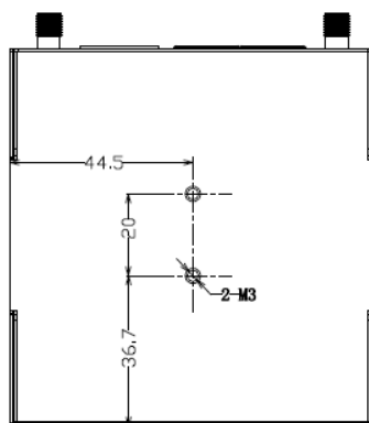
DIN Rail installing position
